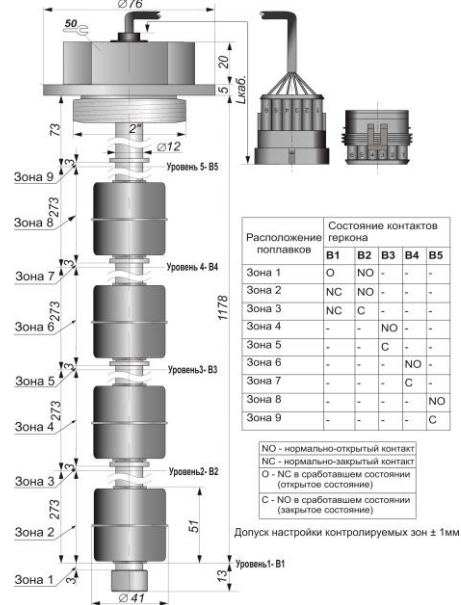
Габаритный чертеж
