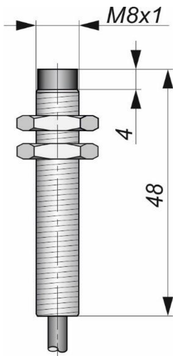
Габаритный чертеж
