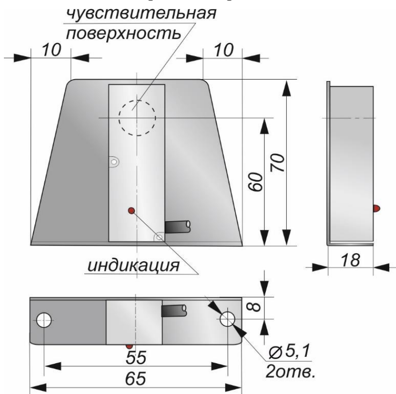
Габаритный чертеж
