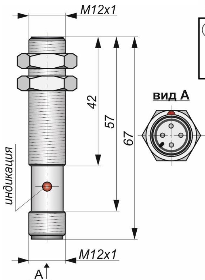
Габаритный чертеж
