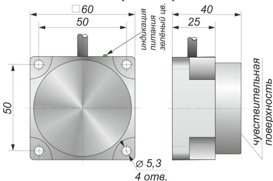
Габаритный чертеж
