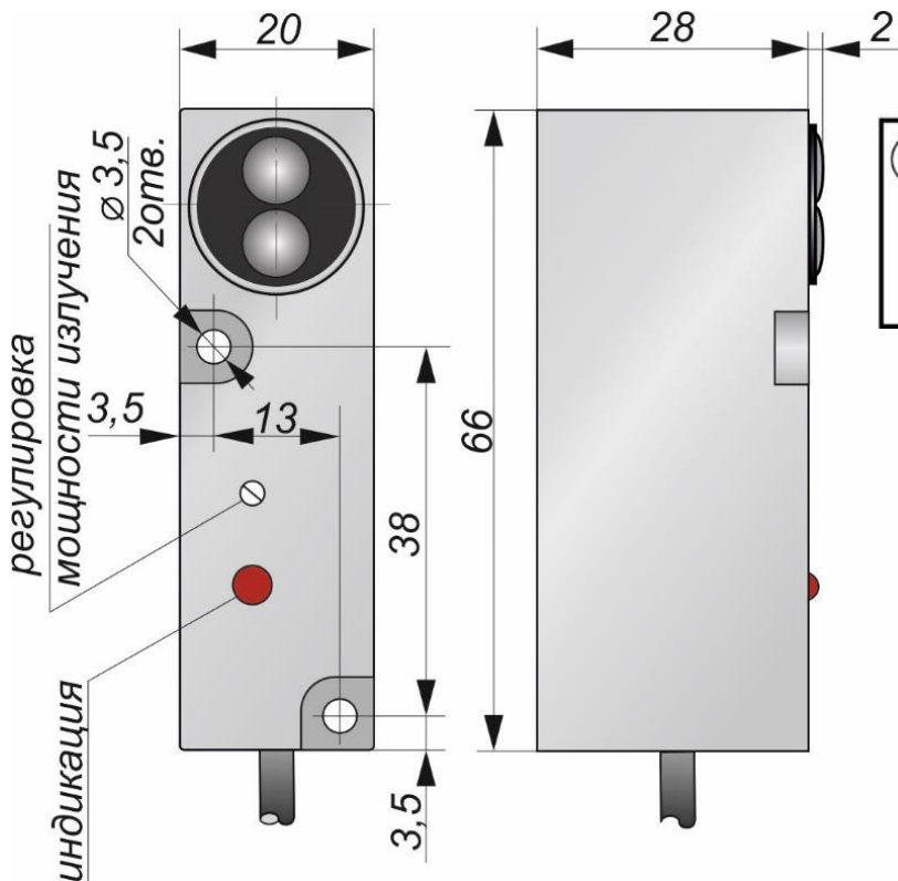
Габаритный чертеж
