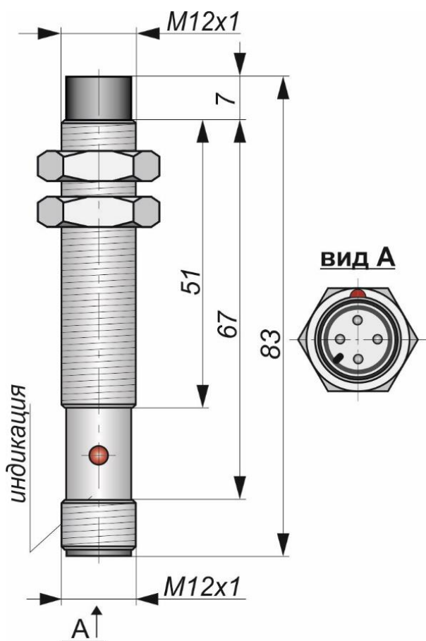
Габаритный чертеж
