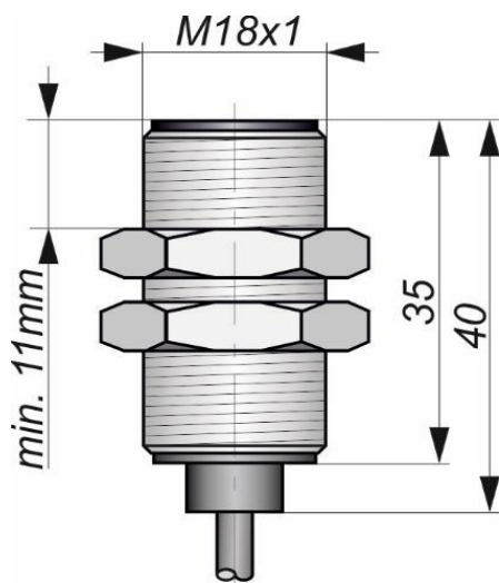
Габаритный чертеж
