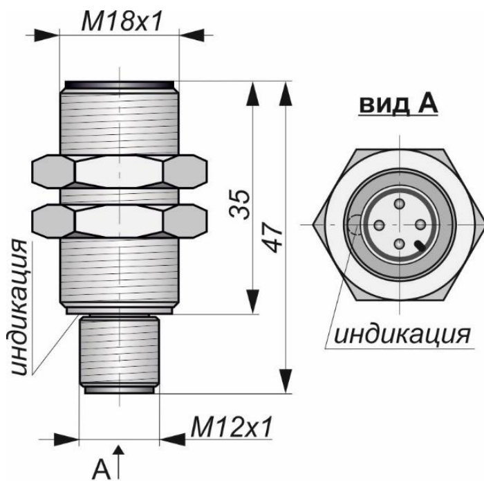
Габаритный чертеж
