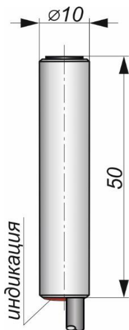
Габаритный чертеж
