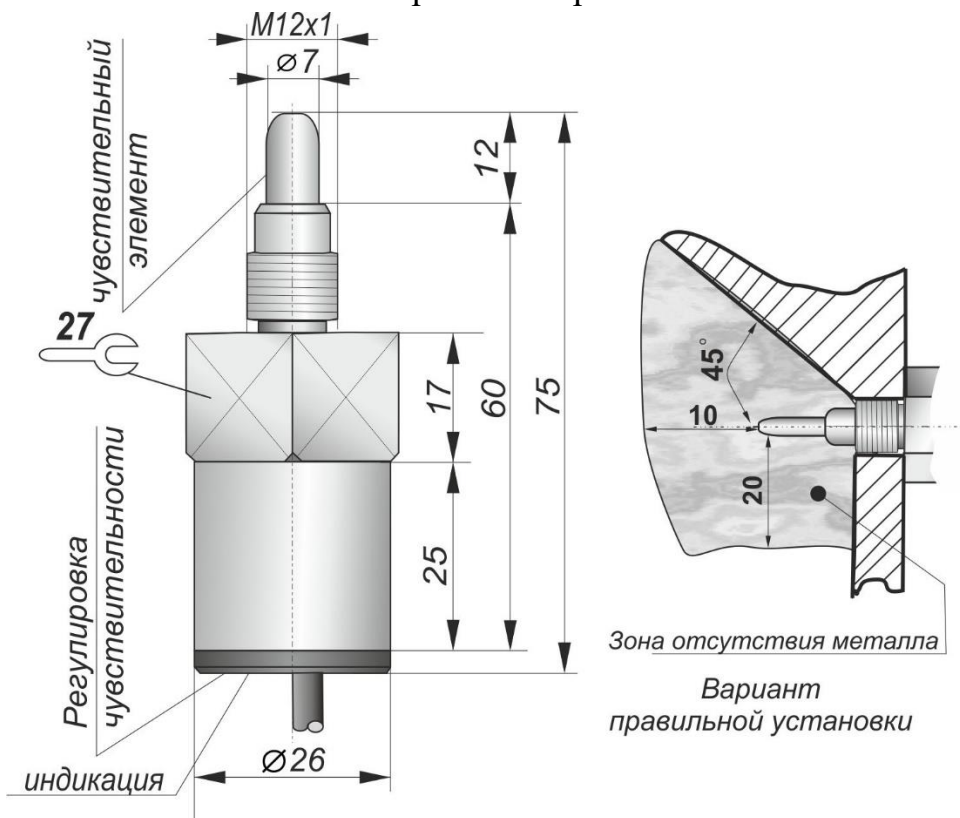
Габаритный чертеж
