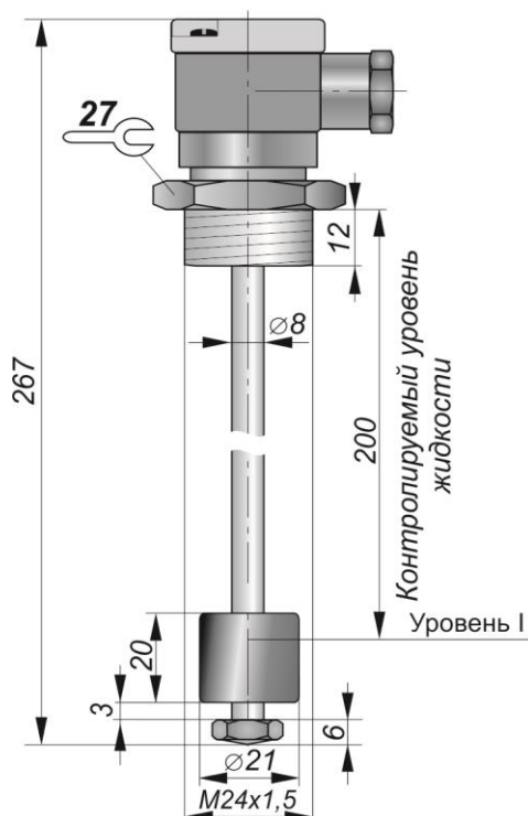
Габаритный чертеж
